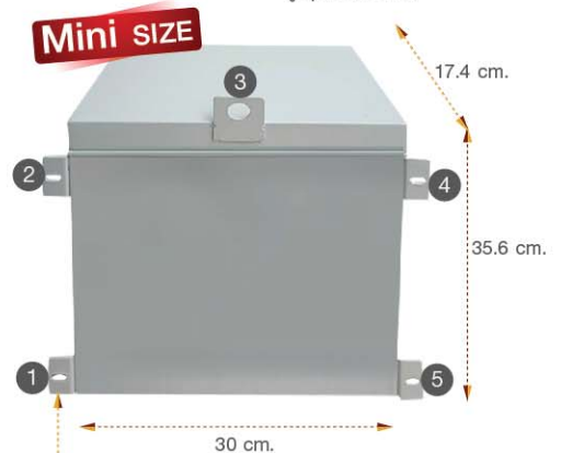
หลังคาติดตั้งพัดลมระบายอากาศ 4 นิ้ว สูงสุดจำนวน 1 ตัว
